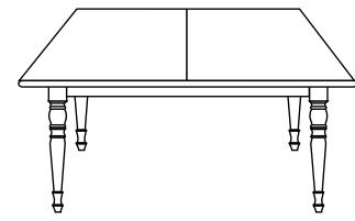
Art. 552/A Tavolo a libro l. 120 p. 70 b. 78 (aperto cm 120x140)
