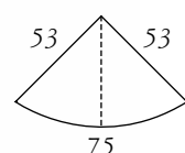
Art. 2136/A Angolo 1p. 1c. lato 53 b. 108
